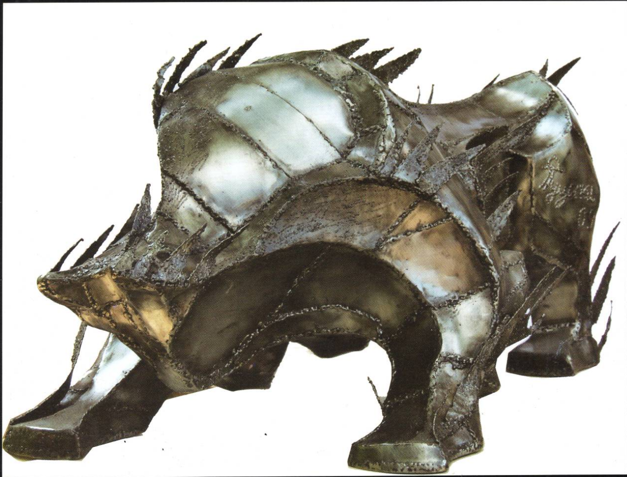
- УРАНСКА СИЛА I (МЕТАЛ) - 55x120x60 cm - 2009 - URAN'S POWER I (METAL) - 55x120x60 cm - 2009
