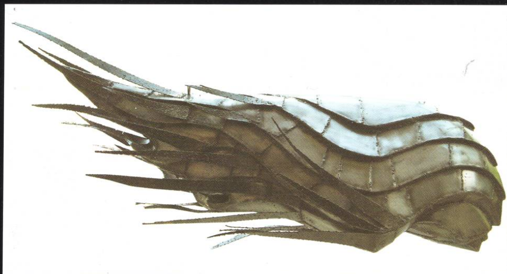
- ПРОСВЕТЛЕНИЕ НА СОВРШЕНСТВОТО I (МЕТАЛ) - 50x150x50 cm - 2009
